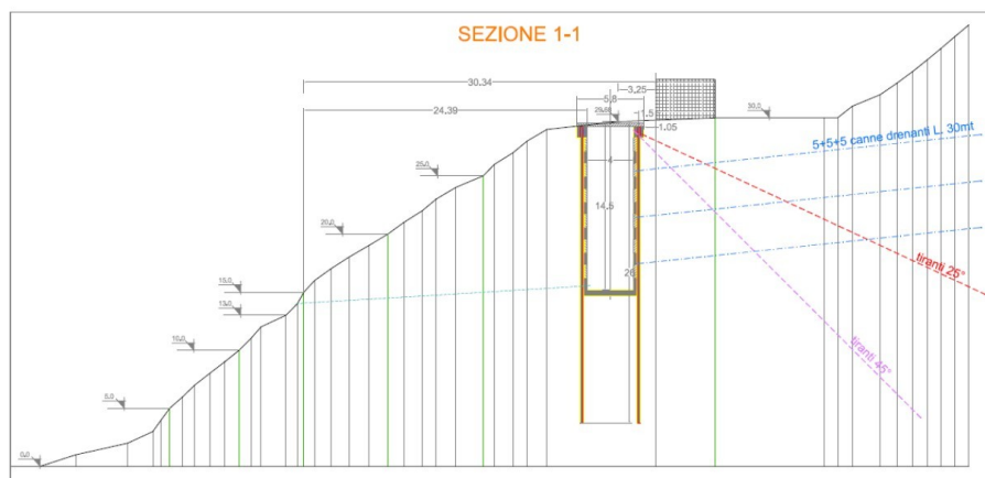
Schema intervento
